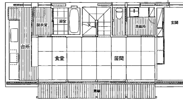
平面図・1階(1/200)
